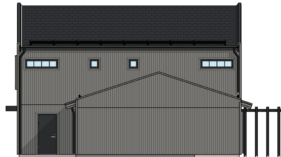
FASAD HÖGERSIDA
