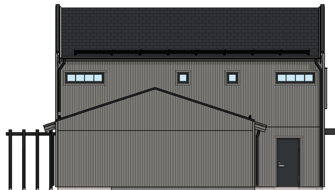
FASAD VÄNSTERSIDA
